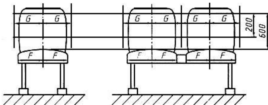
Рисунок Б.1 - Размеры мест сиденья
