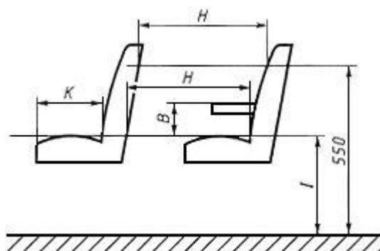
Рисунок Б.2 - Расположение сидений
